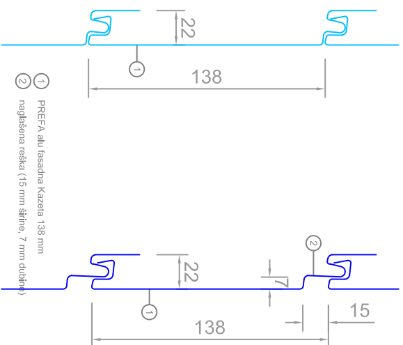
PREFA alu fasadne Kazete širina elementa 138 mm x 0,7mm
