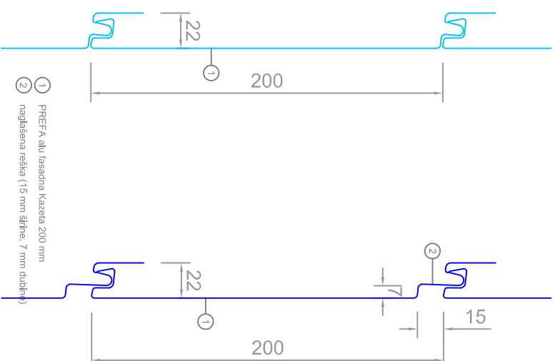
PREFA alu fasadne Kazete širina elementa 200 mm x 1,0mm
