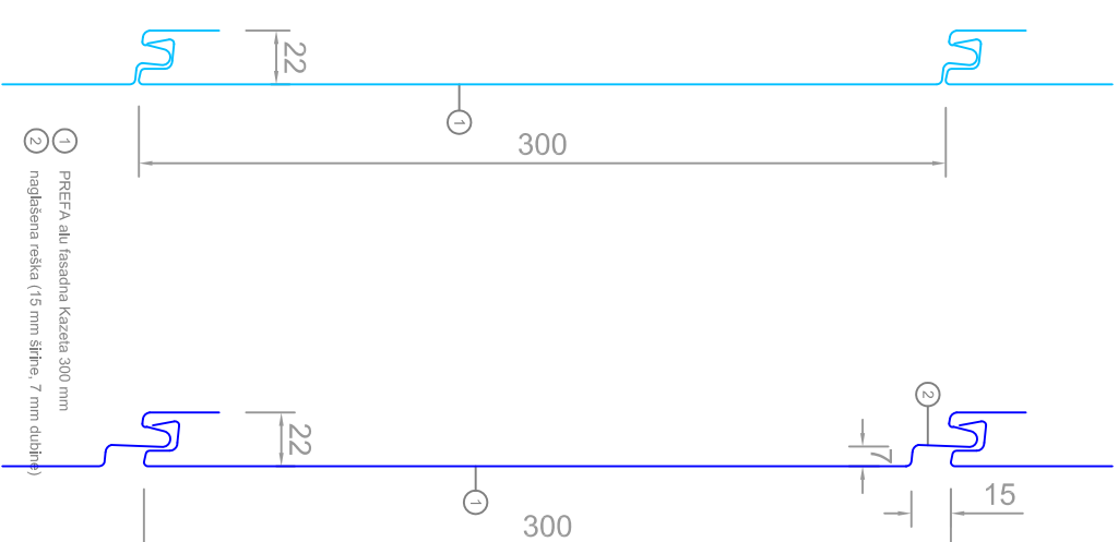
PREFA alu fasadne Kazete širina elementa 300 mm x 1,2mm
